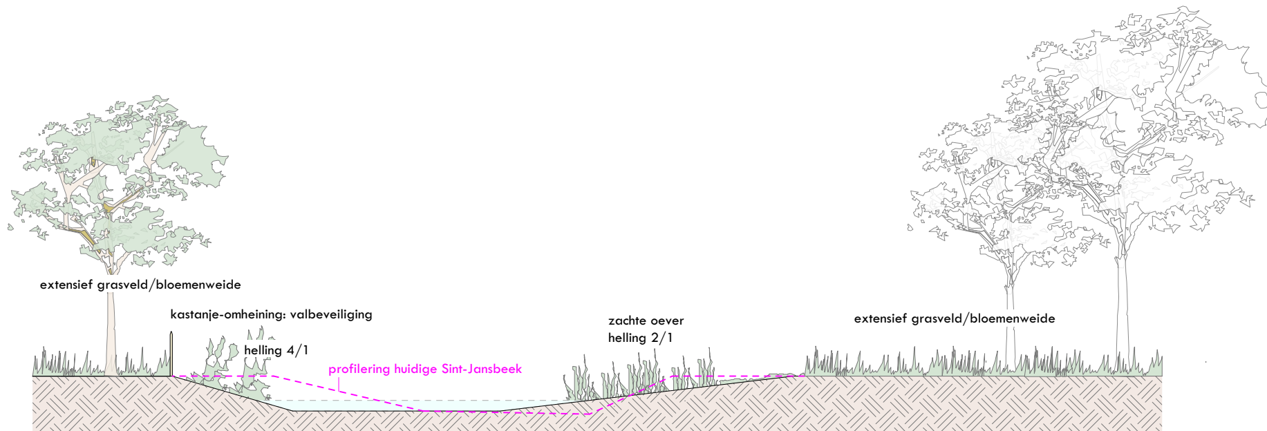
Doorsnede BB
